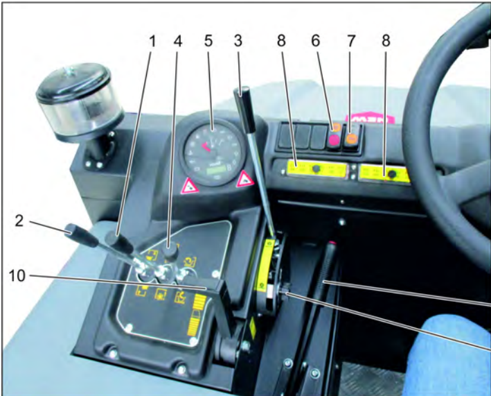
清扫机图片
