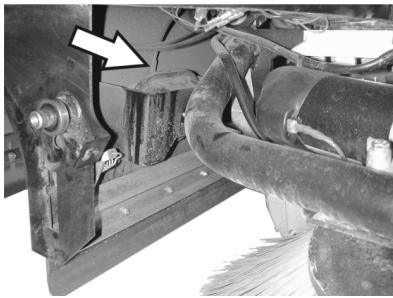
Przyłącze węża do puszki podciśnieniowej mechanizmu opuszczania miotły bocznej
