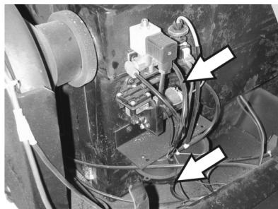
Przyłącza węży do pompy podciśnieniowej i puszki podciśnieniowej (zbiornik)
