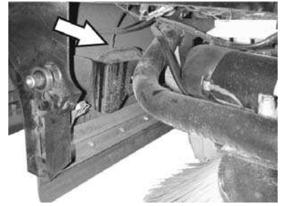
وصلة خراطيم إلى وحدة تفريغ خاصة بإزالة المكثسة الجانبية
