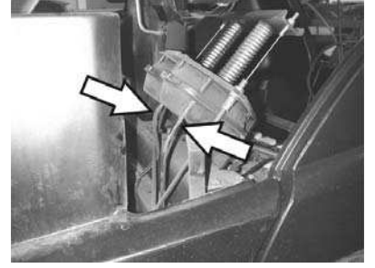
وصلات خراطيم إلى وحدة تفريغ خاصة بإزالة بكرة الكنس
